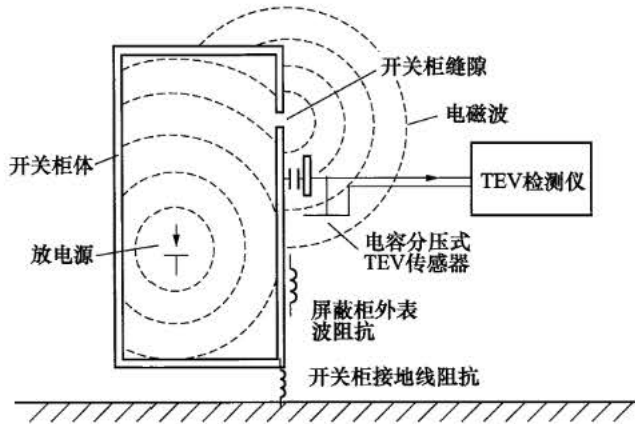
a) 检测原理图
